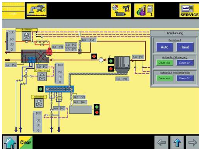
Panel del secador
